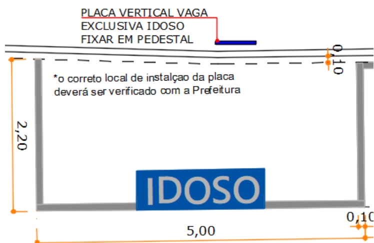
Detalhe pintura da vaga no piso
