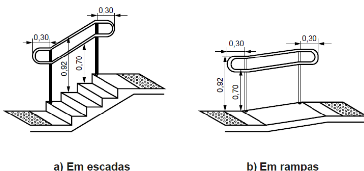
Desenho ilustrativo de corrimão em escada e rampa com prolongamento de 30cm
